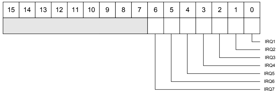
Fig. 2.7: IRQ Status register
