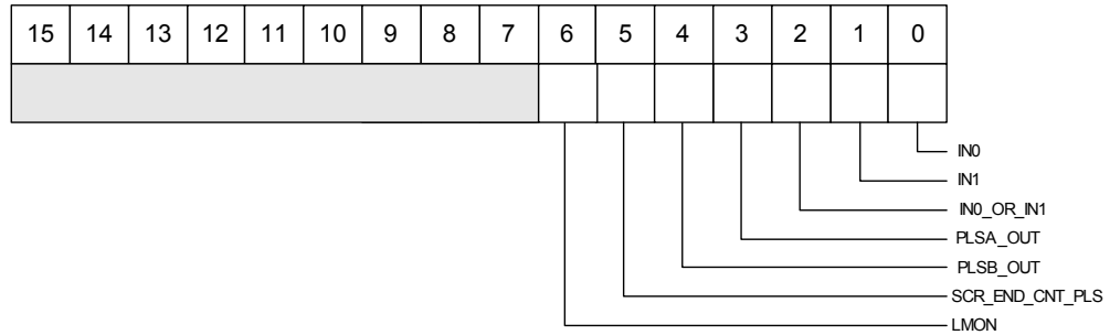
Fig. 2.9: Input register
